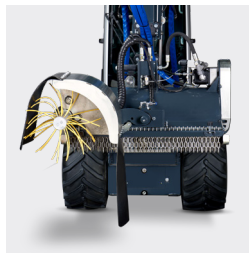
Stockräumbürste (auf Anfrage: individuell steuerbare Bürste)
