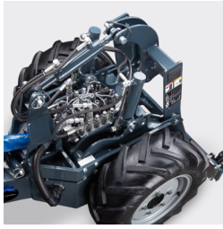
Hydraulikblock mit 1 freien Zylinder für zusätzliche Zylinderbewegungen
